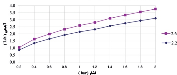
نمودار میزان جریان بر حسب فشارهای مختلف
